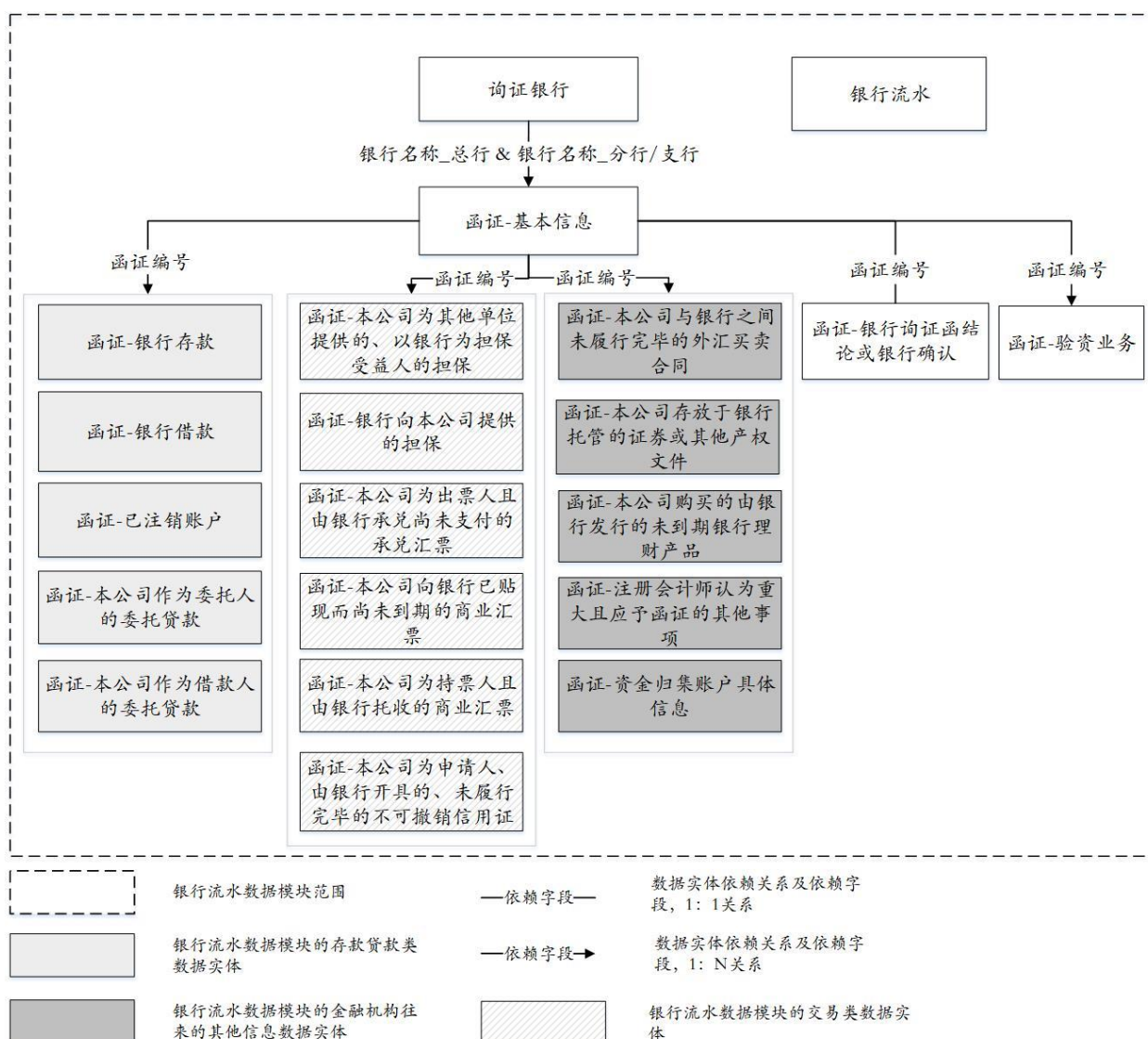
图1 银行流水数据实体关系图
